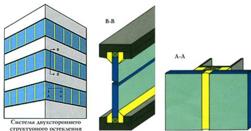
Рис. 36. Стоечно–ригельный фасад со структурным остеклением. Двухстороннее крепление.
