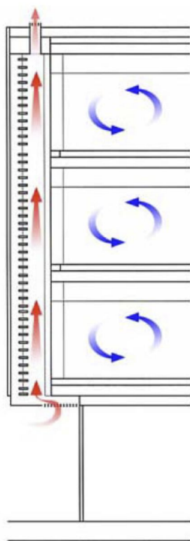
Рис. 58. «Buffer System» (буферная система).
