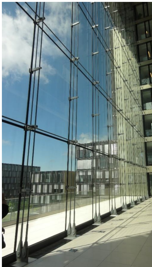
Рис. 51. Вантовое остекление. Thyssen–Krupp–Quartier–Essen–Q1.
