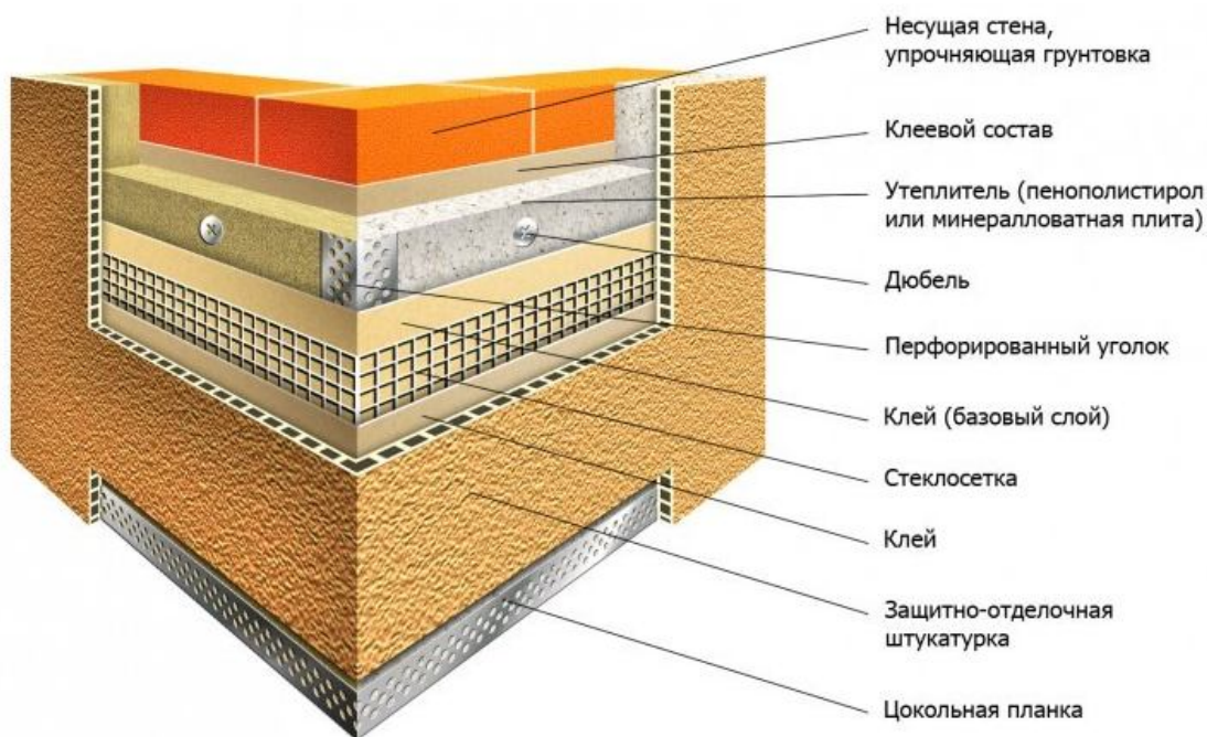
Рис. 5. Штукатурный фасад.
