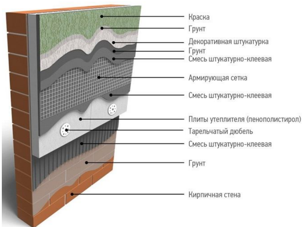
Рис. 6. Схема фасада с тонким штукатурным слоем.
