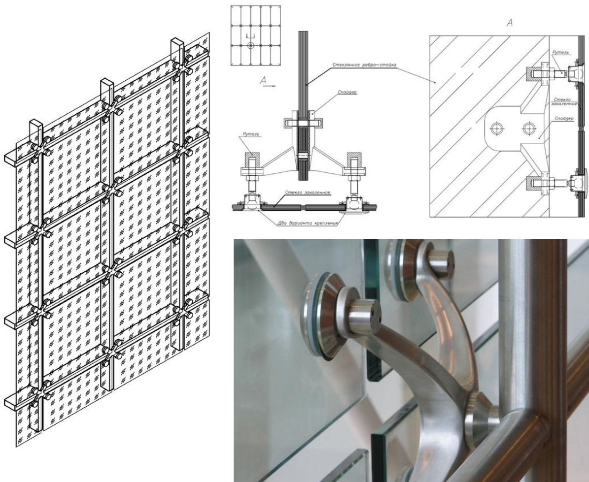
Рис. 46. Спайдерное остекление.
