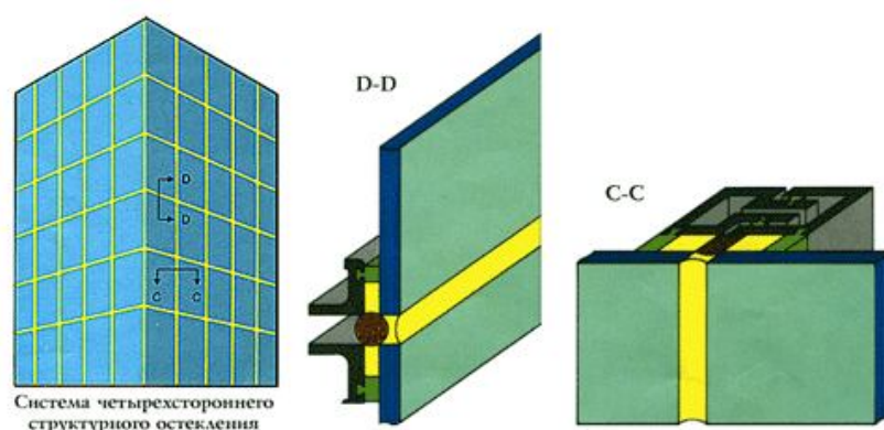
Рис. 37. Стоечно–ригельный фасад со структурным остеклением. Четырёхстороннее крепление.
