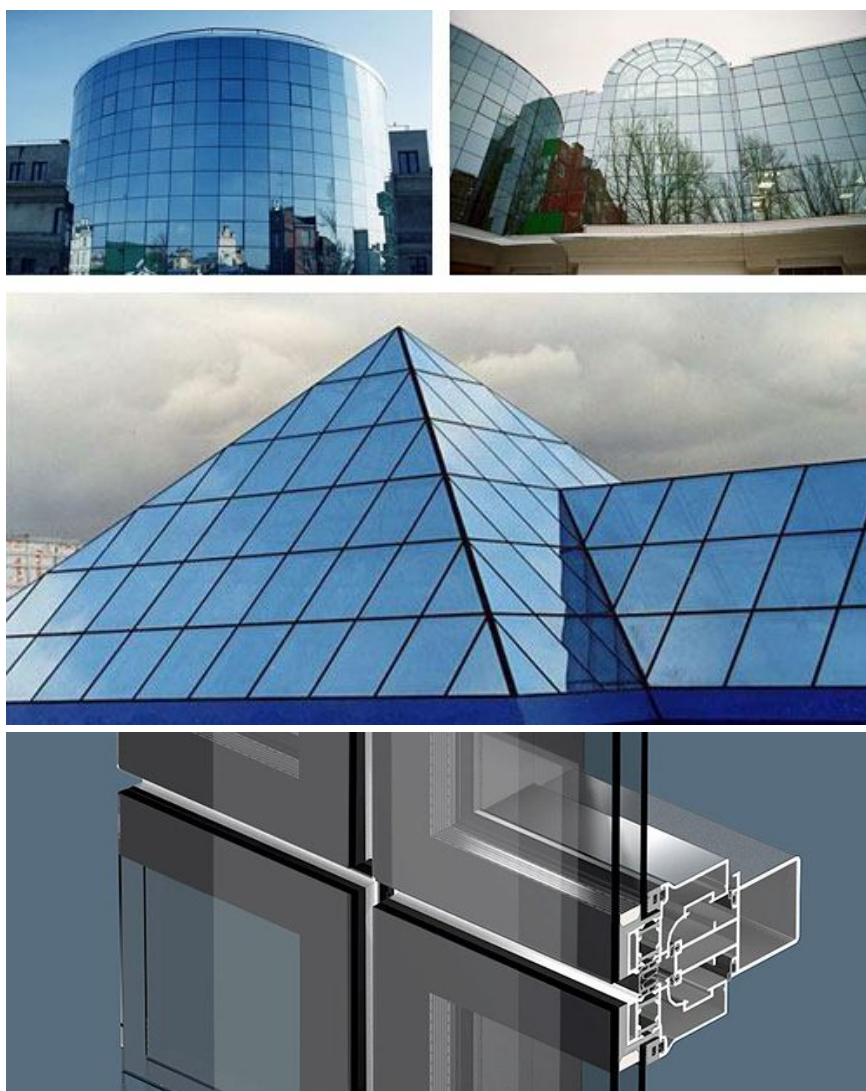
Рис. 34. Стоечно–ригельный фасад со структурным остеклением.
