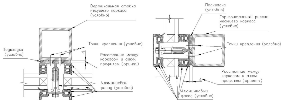
Рис. 43. Алюминиевый фасад по несущему каркасу.
