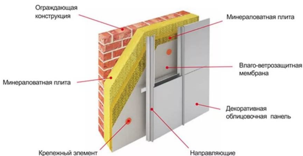
Рис. 10. Схема фасадной системы с вентилируемым воздушным зазором.
