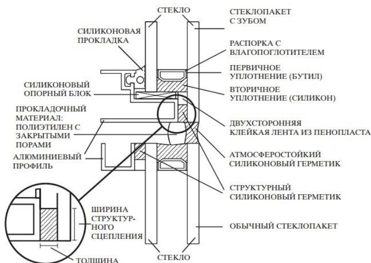
Рис. 38. Стоечно–ригельный фасад со структурным остеклением (вариант секлопакета со стеклами разного размера).
