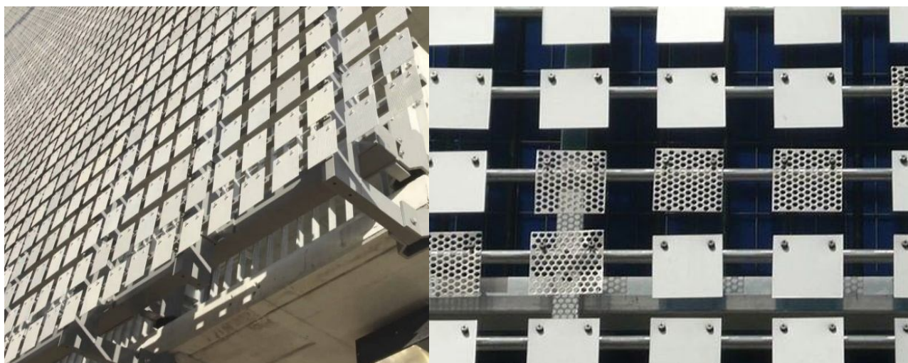
Рис. 23. Алюминиевый фасад паркинга в аэропорте Брисбена, Австралия.
