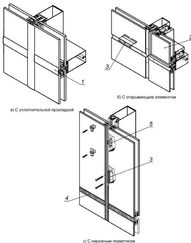
Рис. 35. Стоечно–ригельный фасад со структурным остеклением: 1 – уплотнительная прокладка; 2 – открывающийся элемент; 3 – стеклодержатель; 4 – герметик; 5 – косточка.
