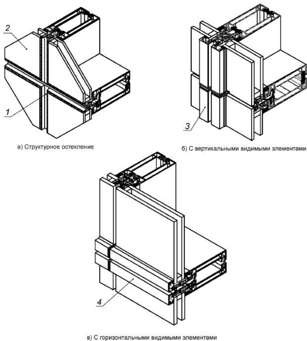
Рис. 41. Модульный фасад структурного и полуструктурного остекления: 1 – уплотнитель; 2 – стеклопакет; 3 – вертикальный видимый элемент крепления; 4 – горизонтальный видимый элемент крепления.
