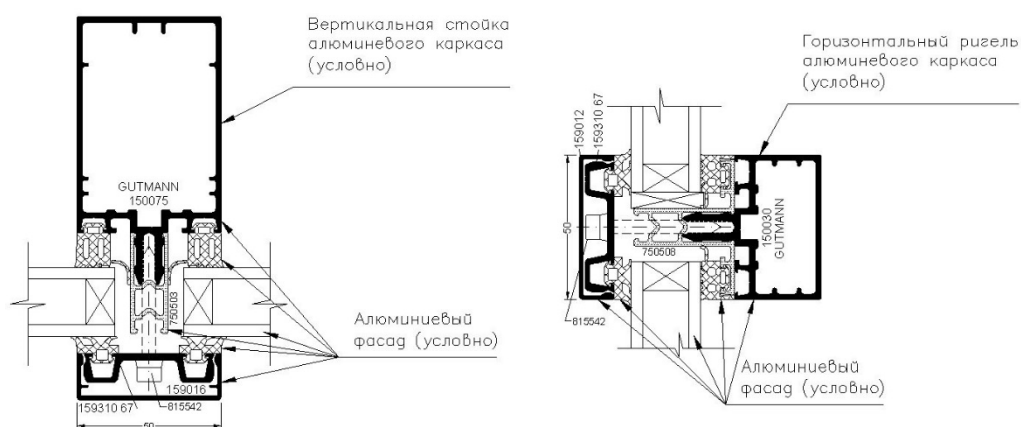
Рис. 42. Самонесущий алюминиевый фасад.
