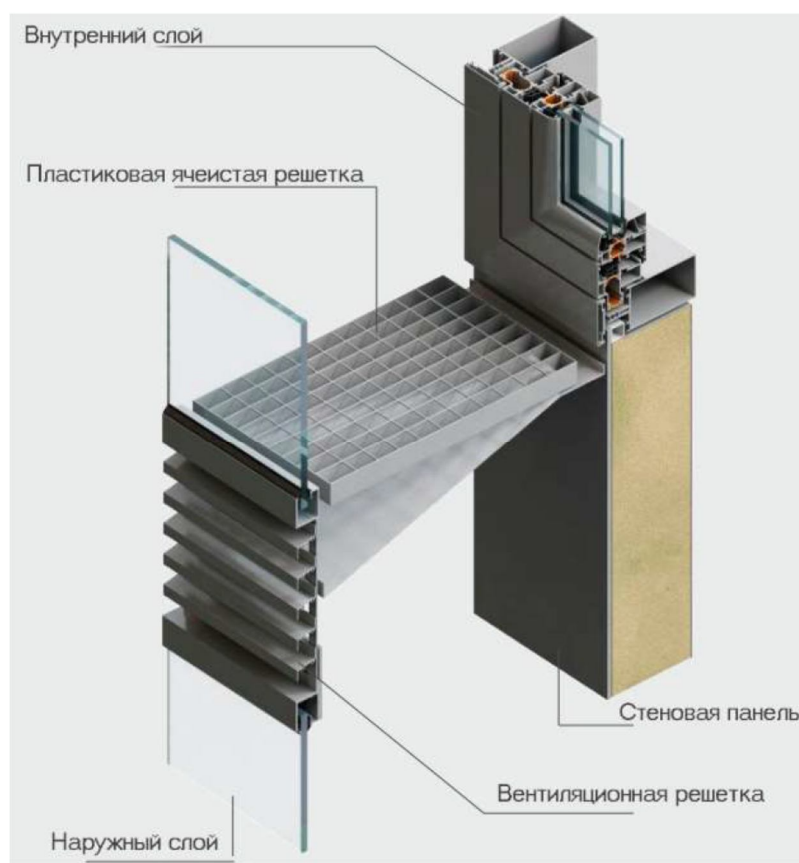
Рис. 54. Конструкция двойного фасада «Double Skin»
