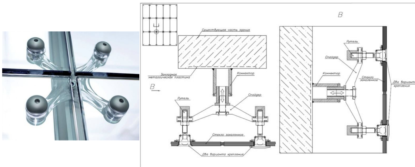
Рис. 49. Спайдерное остекление фасада. Крепление стекла.
