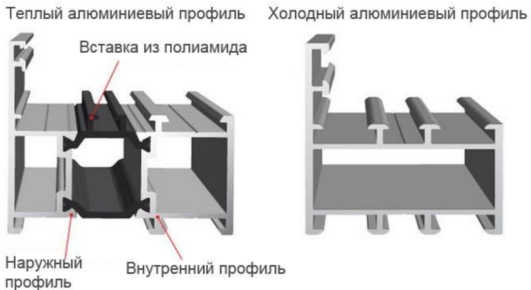
Рис. 4. «Тёплый» и «холодный» алюминиевый профиль.
