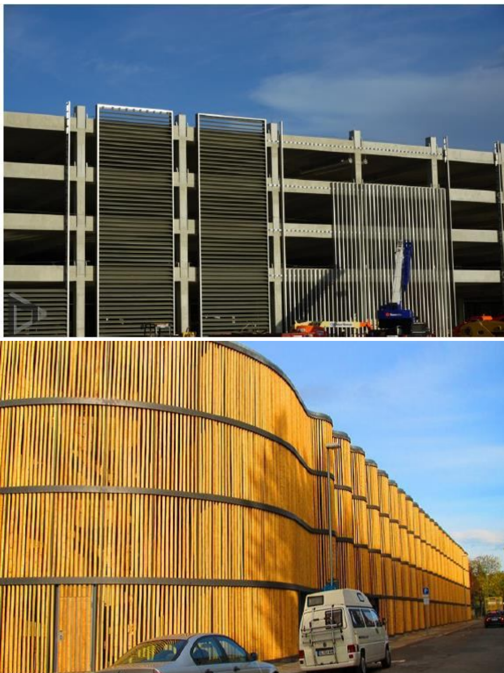
Рис. 20. Фасад жалюзи. Горизонтальное и вертикальное расположение реек на фасаде паркинга. Фасад жалюзи на скруглённых поверхностях.
