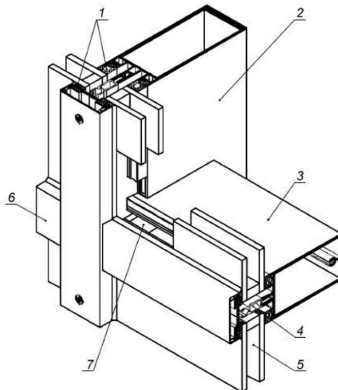
Рис. 33. Стоечно–ригельный фасад рамного остекления: 1 – уплотнитель стекла; 2 – стойка; 3 – ригель; 4 – термоизоляционная вставка; 5 – стеклопакет; 6 – декоративная накладка; 7 – подкладка под стеклопакет
