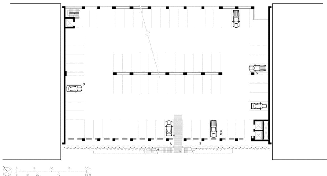
Рис. 64. Гараж в Санта–Монике, США. Архитектурное бюро Behnisch Architekten, 2013.
