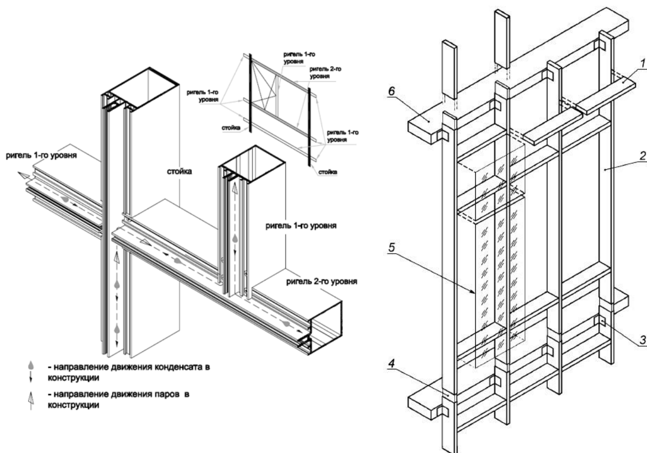
Рис. 28 Стоечно–ригельная светопрозрачная фасадная система из алюминиевого профиль (схема): 1 – ригель; 2 – стойка; 3 – кронштейн; 4 – деформационный соединитель; 5 – светопрозрачное заполнение; 6 – несущий остов здания (междуэтажные перекрытия).
