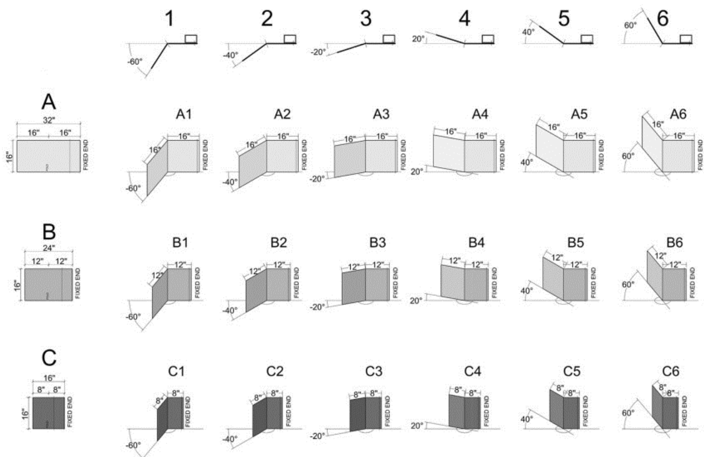
Рис. 25. Фасадные алюминиевые панели.
