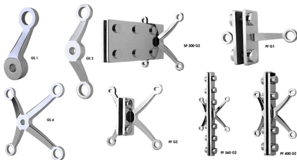
Рис. 45. Крепёжные элементы спайдерного остекления
