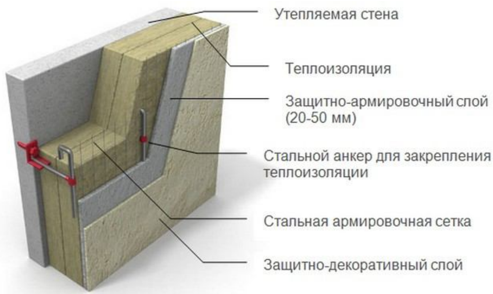
Рис. 8. Схема штукатурного фасада с толстым штукатурным слоем.
