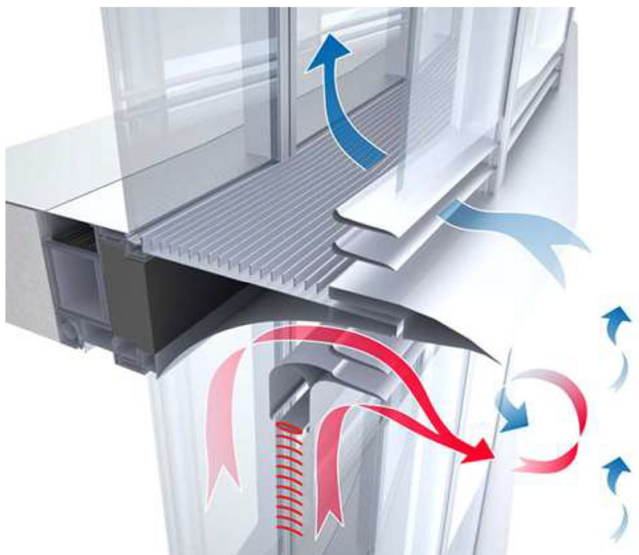
Рис. 57. Вентиляция (поэтажная) двойного фасада «Double Skin»
