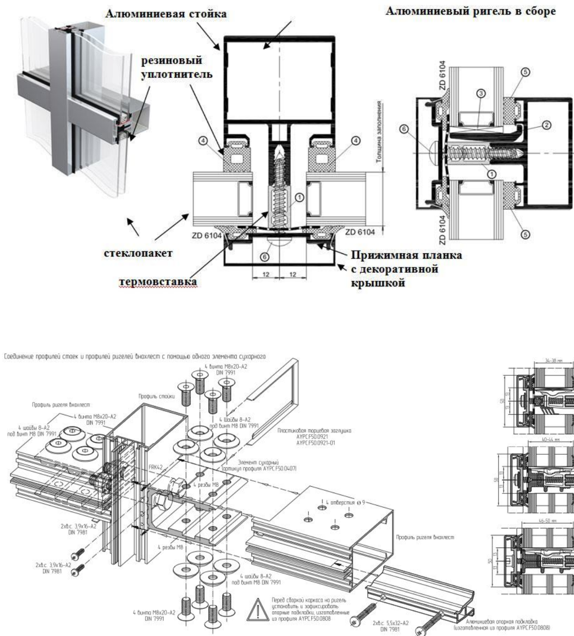
Рис. 30. Стоечно–ригельная светопрозрачная фасадная система из алюминиевого профиля. Узлы.
