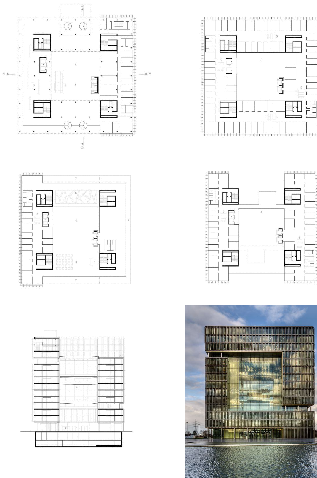
Рис. 52. Thyssen-Krupp-Quartier-Essen-Q1. Планы 1, 2, 3, 7 этажей, разрез. Фасад (фото)
