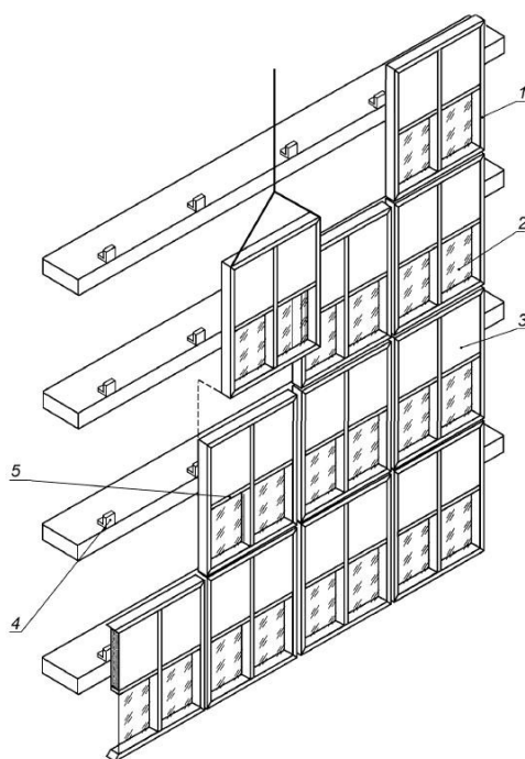
Рис. 40. Модульный фасад (схема): 1 – модульный элемент фасада; 2 – светопрозрачное заполнение; 3 – несветопрозрачное заполнение; 4 – кронштейн; 5 – шпроса.
