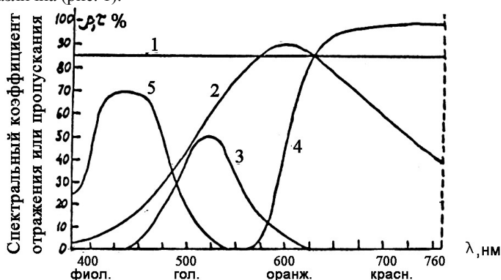
Рис. 1. Кривые спектрального отражения поверхности свежевыпавшего снега (1), желтой бумаги (2) и кривые спектрального пропускания зеленого (3), красного (4) и синего (5) стекол.
