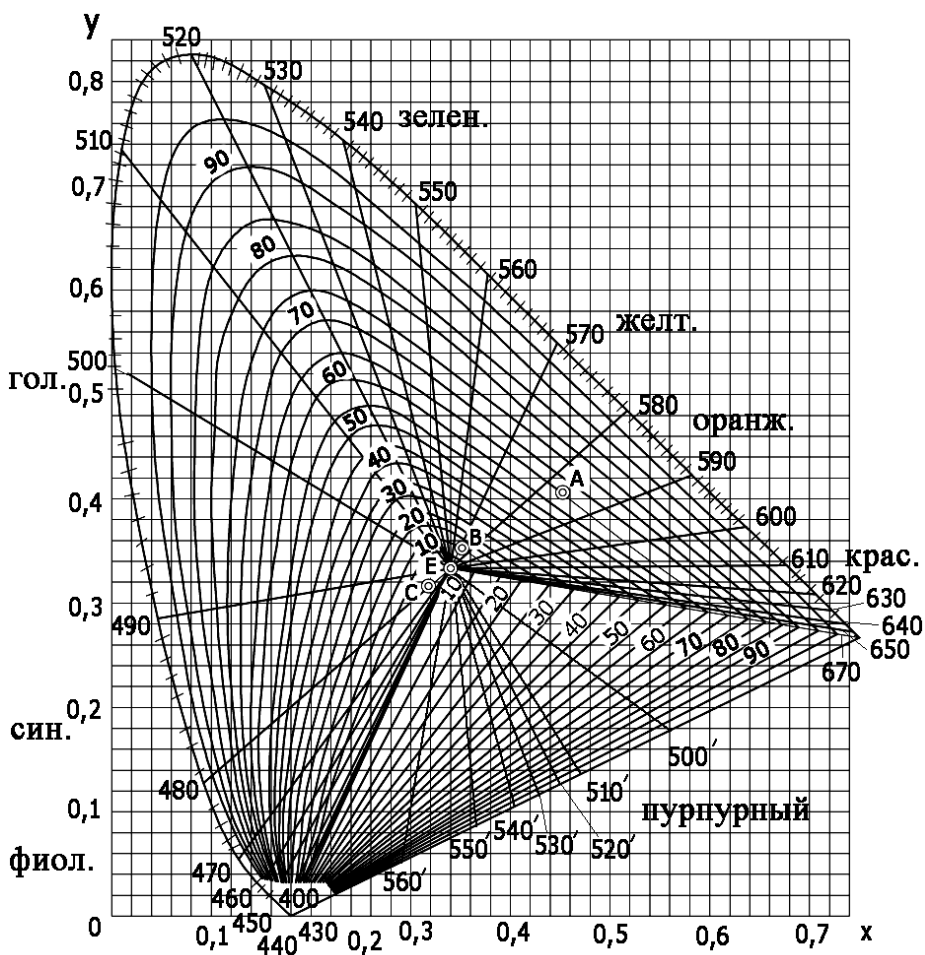
Рис. 10. Диаграмма цветности xу с линиями равной чистоты цвета по отношению к источнику E.
