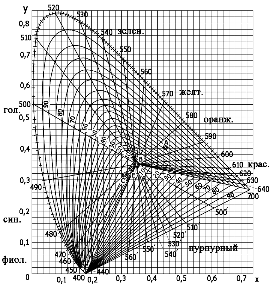
Рис. 8. Диаграмма цветности xy с линиями равной чистоты цвета по отношению к источнику В.
