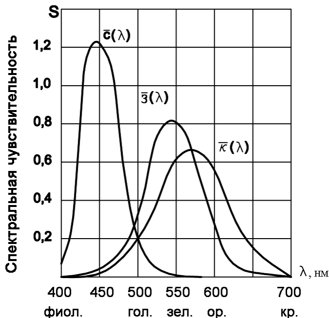
Рис. 2. Спектральная чувствительность цветовоспринимающих КЗС – рецепторов глаза.
