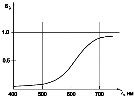
Рис. 12. Спектральный коэффициент отражения оранжевой поверхности.
