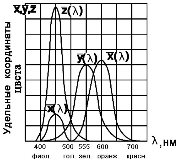
Рис. 5. Кривые сложения стандартного колориметрического наблюдателя МКО в системе \bar{x}\bar{y}\bar{z} .
