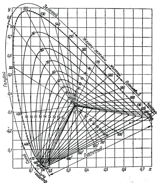
Рис. 11. Цветовой график в международной колориметрической системе.
