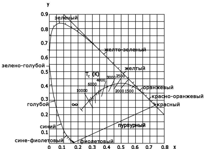
Рис. 4. Цветовой график координат цветности X , Y с линией излучений черного тела и стандартными источниками белого света (A, B, C и D_{65} )
