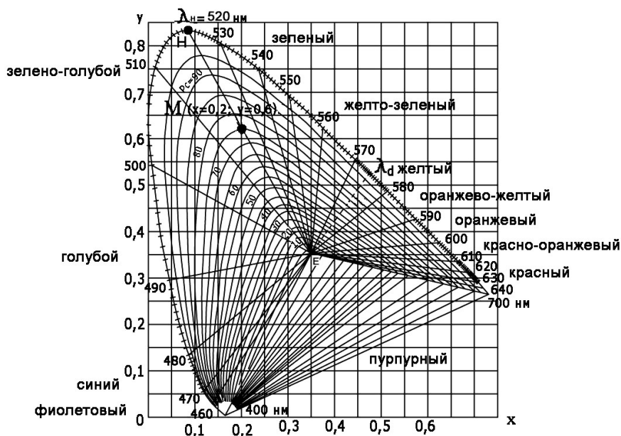
Рис. 11. Определение длины волны и чистоты цвета по диаграмме цветности по отношению к источнику Е.
