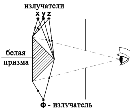
Рис. 3. Схема воспроизведения цвета \Phi смешением трех основных цветов XYZ.
