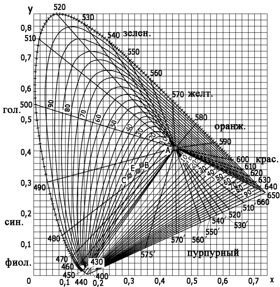
Рис. 7. Диаграмма цветности xу с линиями равной чистоты цвета по отношению к источнику А.
