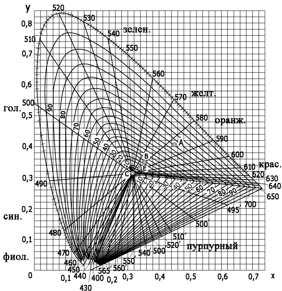
Рис. 9. Диаграмма цветности xy с линиями равной чистоты цвета по отношению к источнику C .
