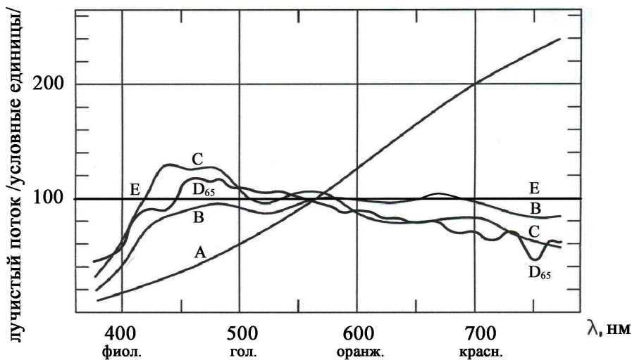
Рис. 6. Относительное спектральное распределение энергии стандартных источников белого света A, B, C, E, D 65 .
