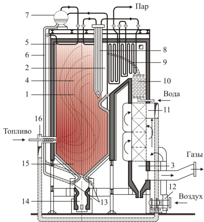
Рис. 48. Схема парового котла в разрезе
