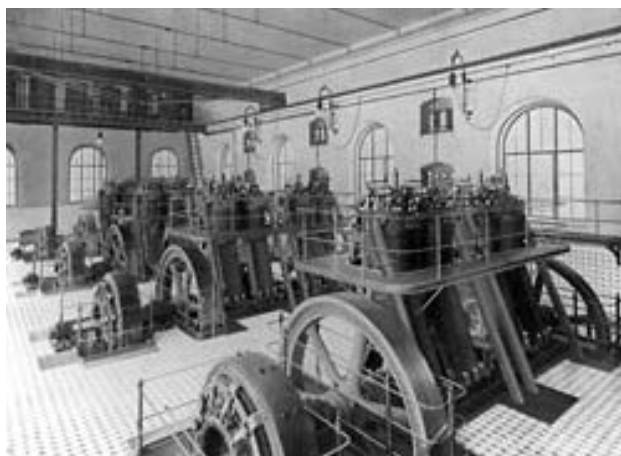
Рис. 15. Первая в России дизельная электростанция "Александровская" в Киеве была оснащена четырьмя дизелями. Введена в строй в 1904 г.
