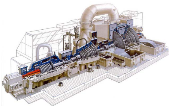
Рис. 64. Паровая турбина в разрезе
