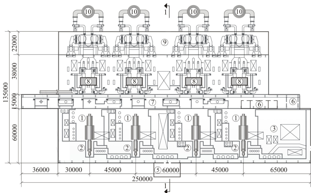
Рис. 38. План главного корпуса ТЭЦ на твёрдом топливе с четырьмя энергоблоками и поперечной компоновкой турбин суммарной мощностью 600 МВт на отметке площадки обслуживания
