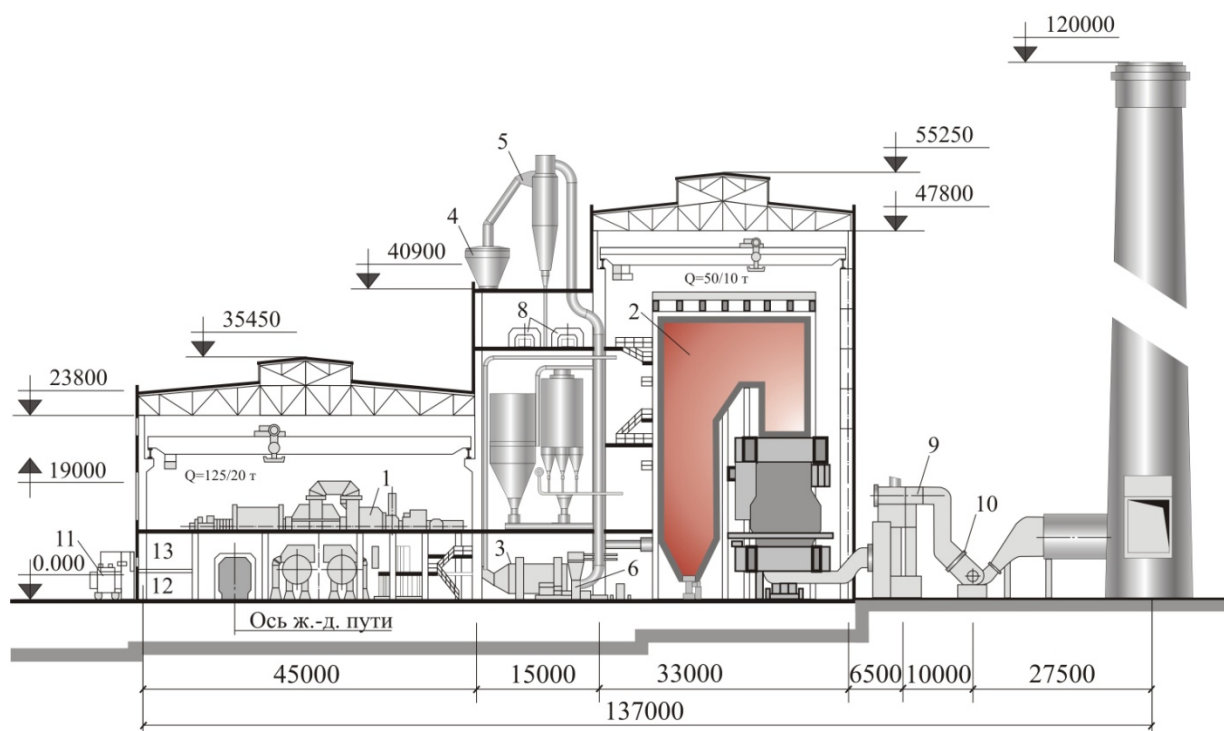
Рис. 35. Поперечный разрез главного корпуса ТЭЦ с тремя энергоблоками на твердом топливе с поперечной компоновкой турбин мощностью 525 МВт
