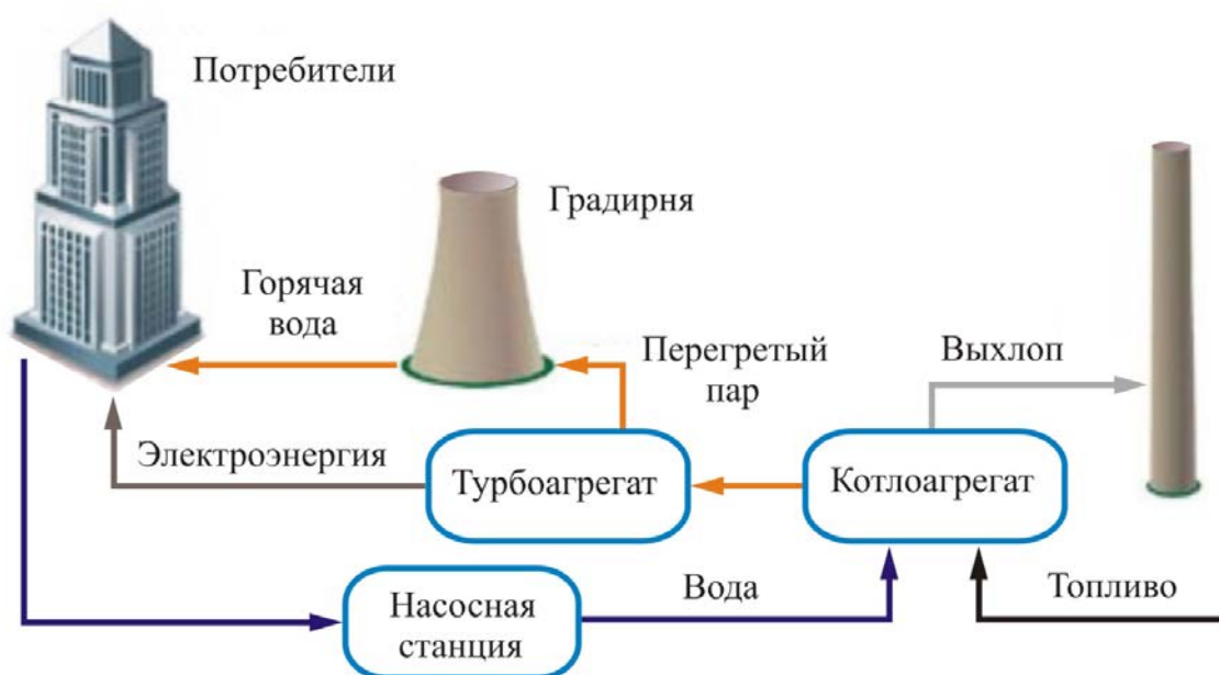
Рис. 4. Принципиальная схема работы ТЭЦ
