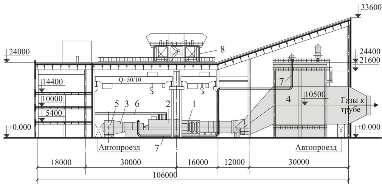
Рис. 42. Поперечный разрез главного корпуса ТЭЦ ПГУ-170 с одновальным расположением турбин
