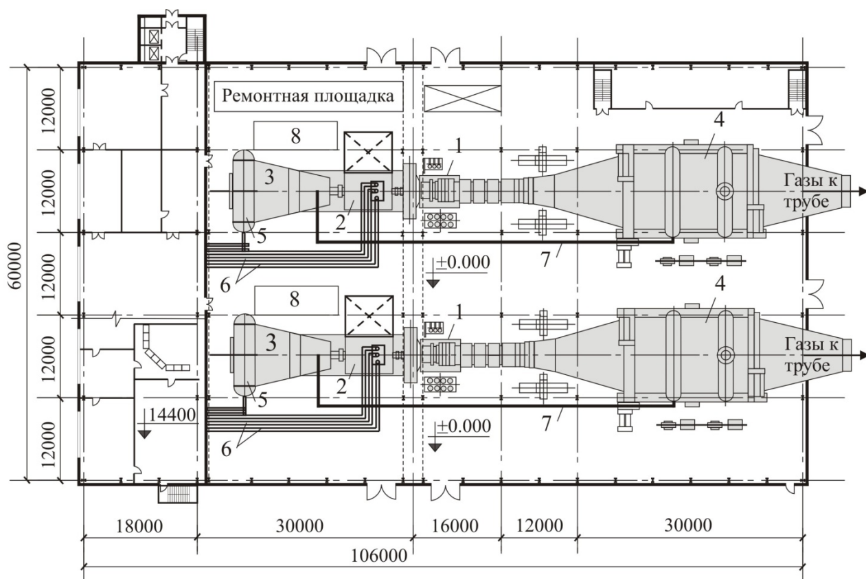
Рис. 43. Компановка плана главного корпуса ТЭЦ ПГУ-170 с двумя энергоблоками
