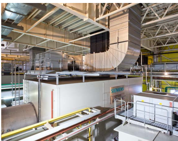
Рис. 106. Воздуховоды
