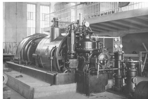
Рис. 13. Ивановская ТЭЦ. Турбина фирмы Круппа
