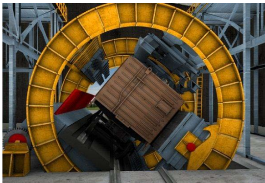
Рис. 61. Роторный вагоноопрокидыватель
