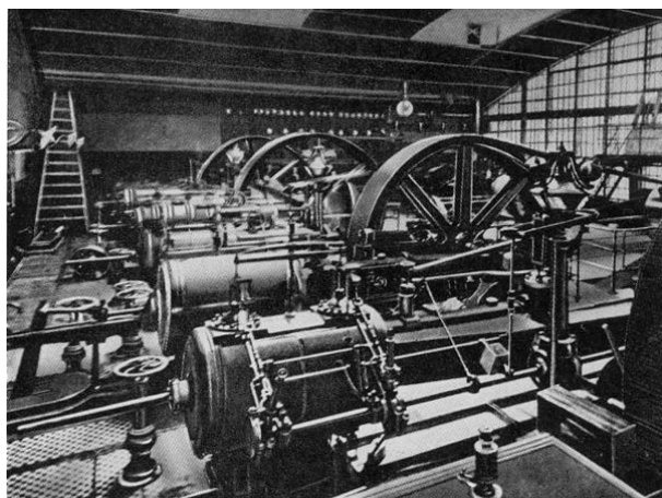
Рис. 14. Электростанция Зимнего дворца. Машинный зал, фото 1901 г. В 1886 году в одном из внутренних дворов Нового Эрмитажа, который с тех пор носит название Электродвор, была построена электростанция по проекту техника дворцового управления Василия Леонтьевича Пашкова. Эта электростанция была крупнейшей во всей Европе на протяжении 15 лет
