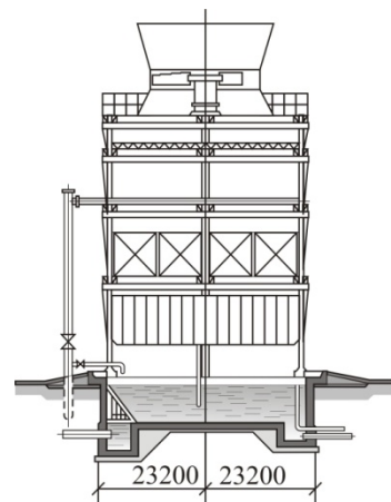
Рис. 70. Вентиляторные секционные эжекторные градирни. Справа – поперечный разрез
