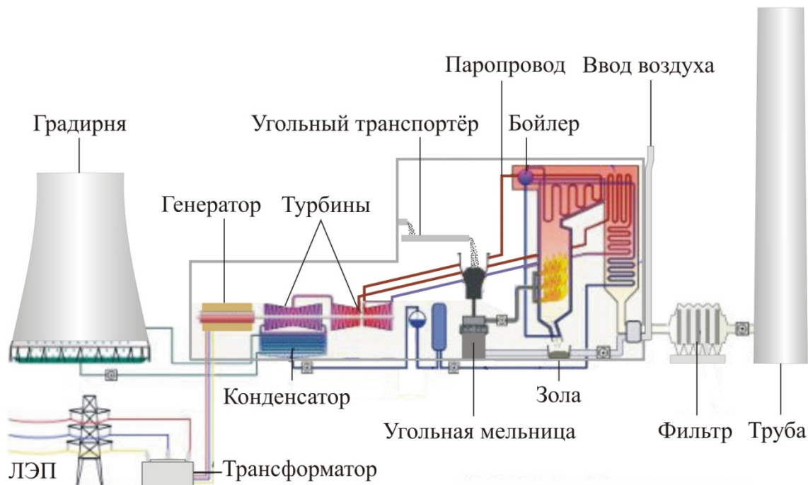
Рис. 1. Технологическая схема КЭС
