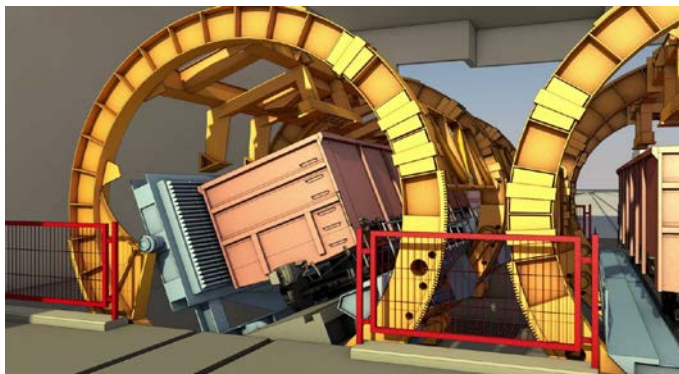
Рис. 61. Роторный вагоноопрокидыватель
