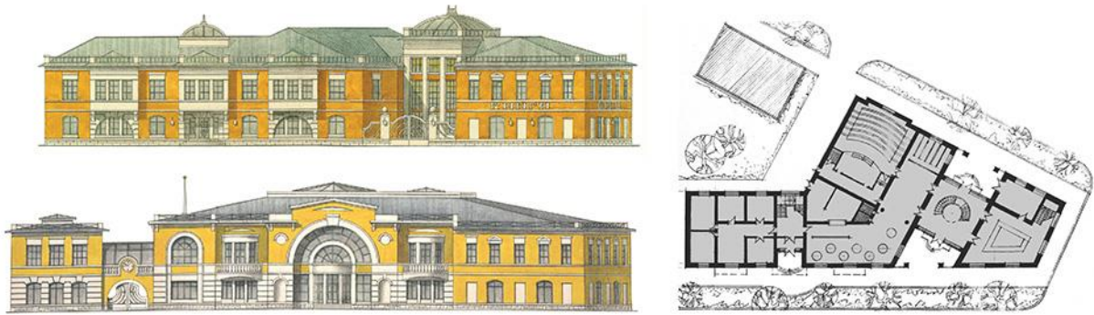
Рис. 5. Проектное предложение по созданию гостинично-прогулочной зоны Левобережья г. Торжка, 2003 г. – культурно-развлекательный центр «Илья» в восстанавливаемом и расширяемом историческом доме № 1а по Ильинской площади, варианты объемно-планировочного решения, план 1 этажа
