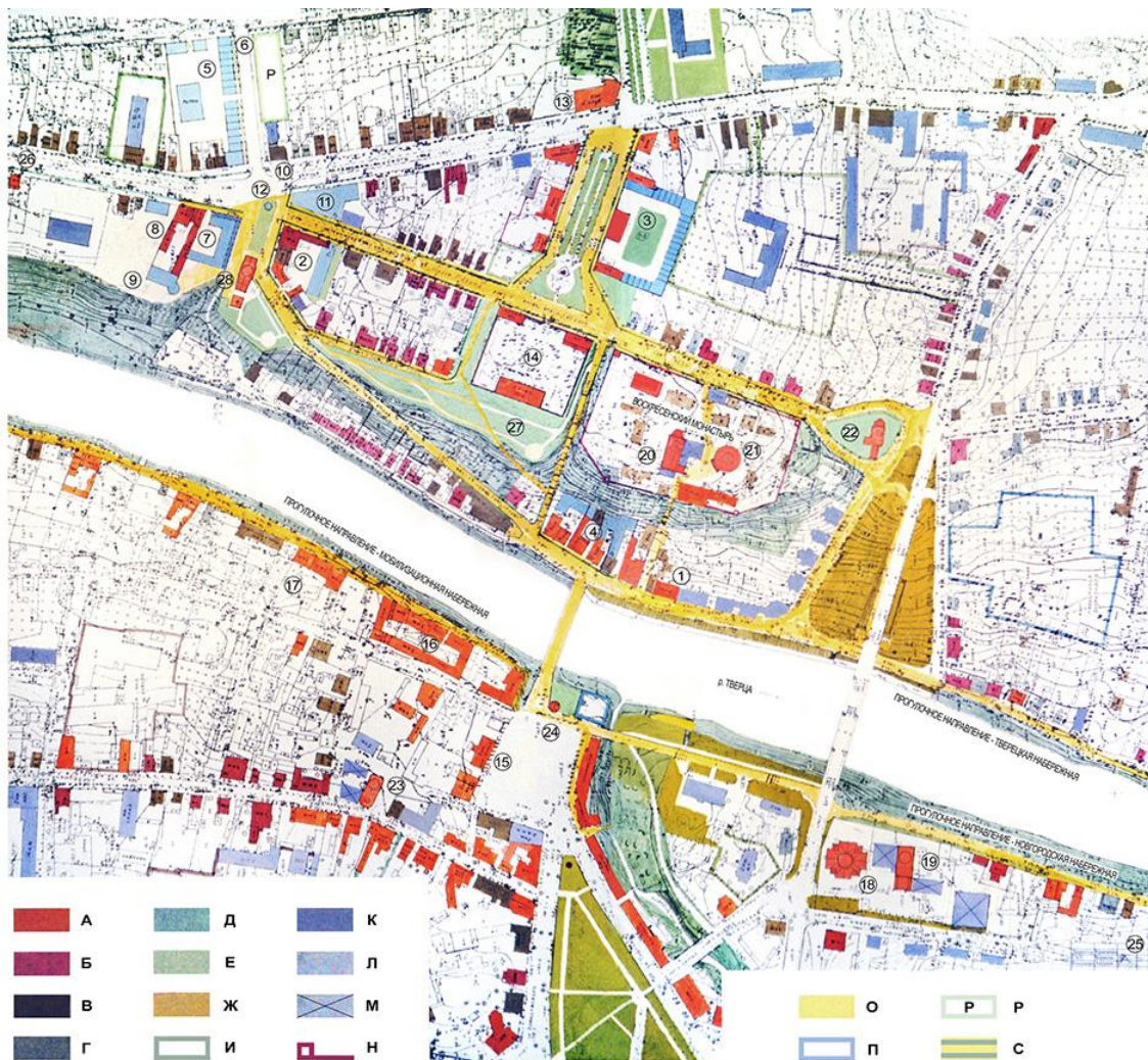
Рис. 4. Проектное предложение по созданию гостинично-прогулочной зоны Левобережья г. Торжка, 2003 г., план-схема планировочной и функциональной организации и благоустройства: 1 – реконструируемая гостиница «Тверца»; 2 – гостиница «Ильинка»; 3 – гостиница и мотель «У Городничего»; 4 – комплекс малых специализированных гостиниц; 5 – Ильинский рынок; 6 – Ильинский пассаж, торговые ряды; 7 – универмаг «Параскева Пятница»; 8 – музей народной артистки России Т.Ф. Тугариновой; 9 – трактир «Ямской»; 10 – муниципальная галерея архитектора Л.В. Андреева; 11 – культурно-
