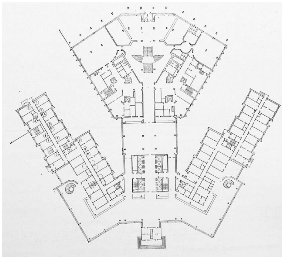
Рис. 12. Гостиница «Салют». План первого этажа
