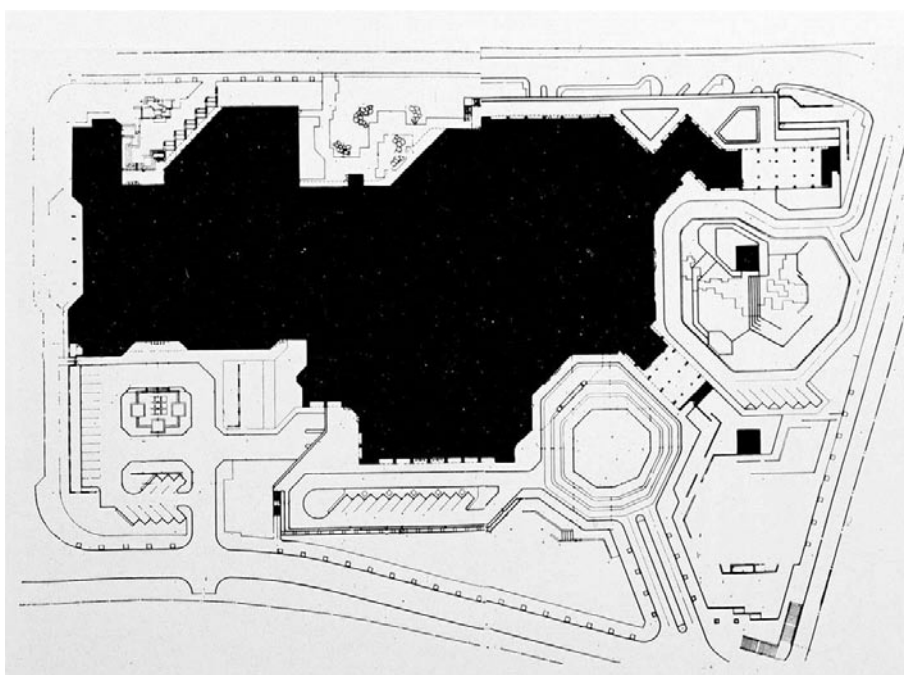
Рис. 16. Центр Международной торговли. Генеральный план участка
