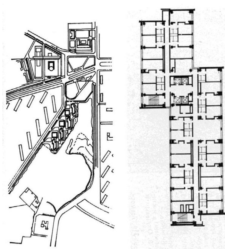
Рис. 10. Гостиница «Севастополь». Генеральный план и план жилого блока
