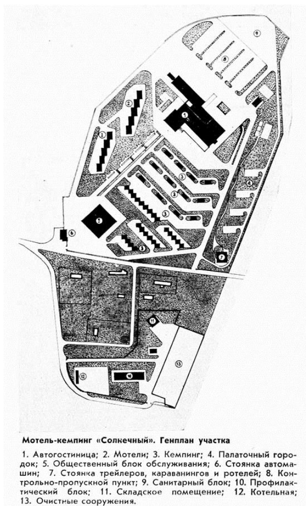
Рис. 14. Мотель «Солнечный». Генеральный план (в настоящее время сохранился только основной корпус, 1 на схеме)
