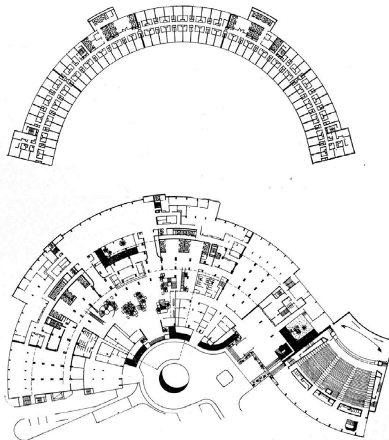
Рис. 9. Гостиница «Космос». План типового и первого этажей
