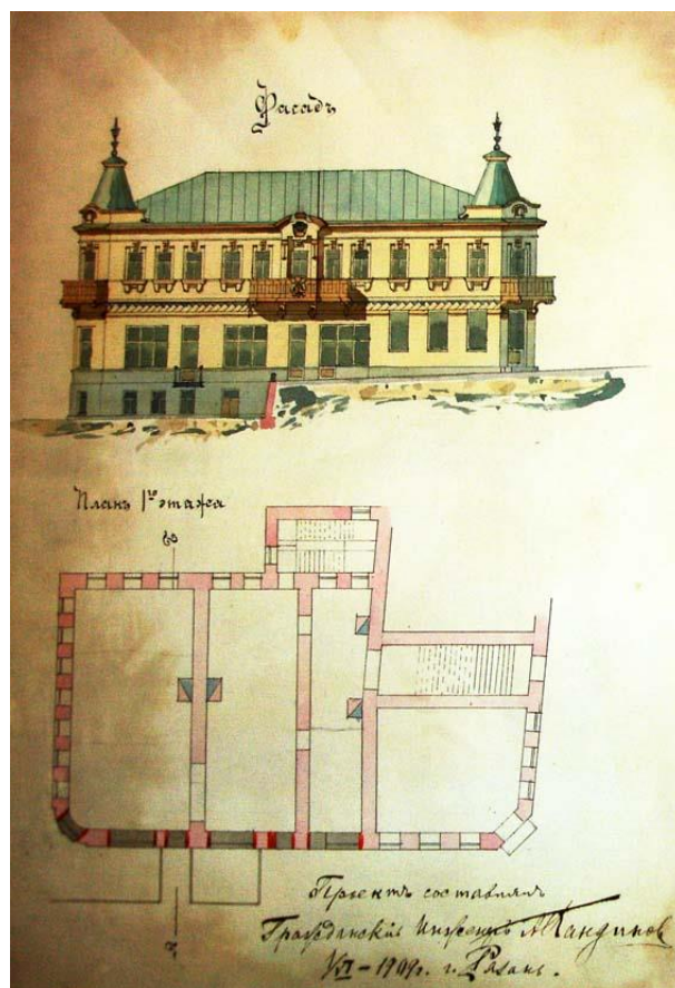
Рис. 7. Фасад и план дома купца Н.А. Рудометкина
