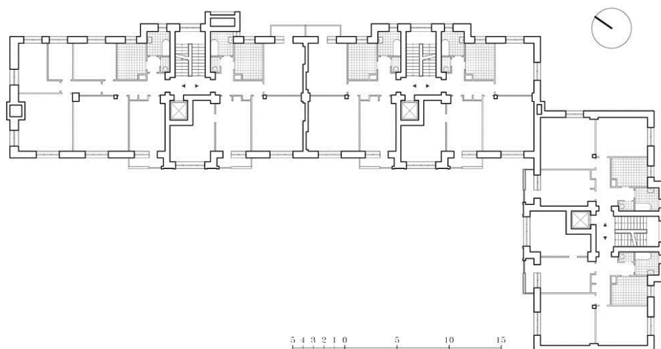
Рис. 2. План 7-го этажа жилого комплекса для сотрудников НКВД в Б. Златоустинском пер. Арх. Л.З. Чериковер, Н.И. Арбузников, 1932-1934 (графическая реконструкция М.Б. Князева по данным БТИ, архитектурным обмерам и др.)
