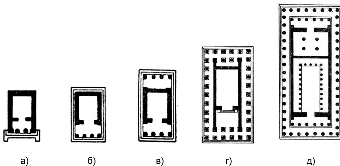
Рис. 5. В истории архитектуры развертывание протяженной храмовой структуры наиболее наглядно представлено еще Витрувием для Античной Греции: от храма в антах (а) до периптера (д) [2]
