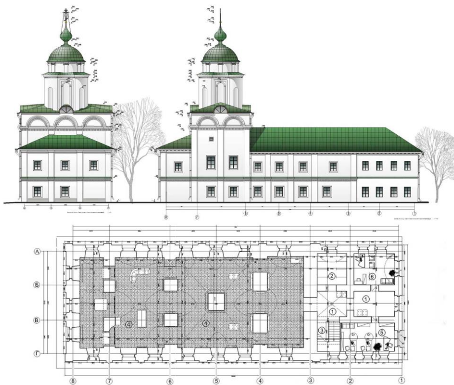
Рис. 2. Церковь Архангела Гавриила Владимирского прихода города Вологды, 1669 г. Северный и восточный фасад (вверху); план подклетного яруса (внизу). Дипломный проект К.А. Разумова (научный руководитель профессор И.К. Белоярская).
