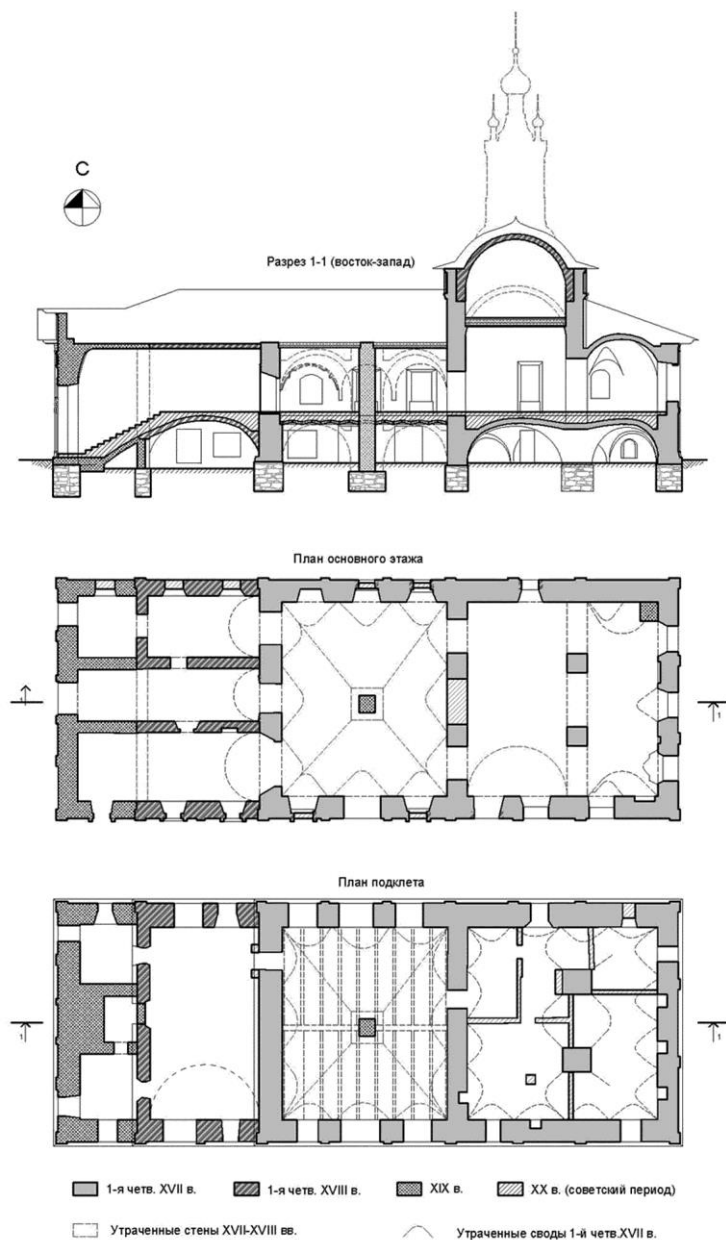
Рис. 10. Схемы трех строительных этапов формирования архитектуры теплого храма Богоявления, определенные в результате проведенных историко-архивных и натурных исследований
