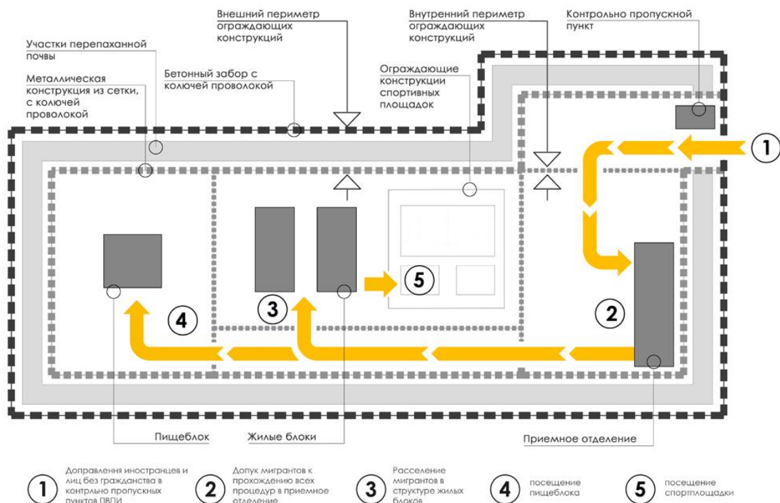
Рис. 8. Схема создания разграничения и ограждающих конструкций ПВПИ в Журавичах, Волынской области
