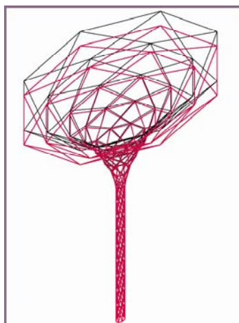
Рис. 5. Гипертрофированная деформация геометрии колонны под нагрузкой
