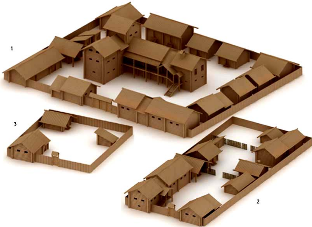
Рис. 1. Реконструкции городских усадеб различных слоев населения: 1) подворье крупного вотчинника; 2) жилой двор молотчего посадского человека; 3) жилой двор бобыля (Реконструкция автора, компьютерная графика студентов С.А. Глубокина, Е.Д. Мурунец, М.З. Стаменковича, В.И. Стебенковой)
