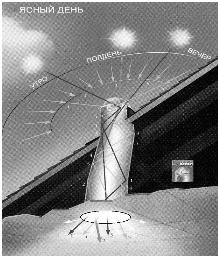
Рис. 19. Схема устройства и действия световода.
