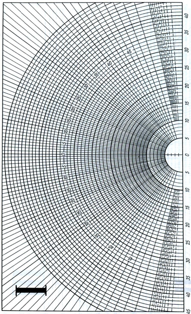
Рис. 36. График І А. М. Данилюка (НИИСФ).
