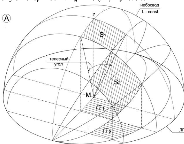
Рис. 30. Деление полусферы равномерно яркого (облачного) небосвода на элементы «равной световой активности» по методу А.М. Данилюка – принципиальная схема, в которой \sigma_1 = \sigma_2 (к закону проекции вектора телесного угла).
