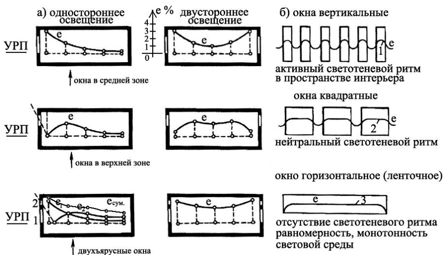
Рис.2. Классификация проемов бокового освещения и типы окон:
