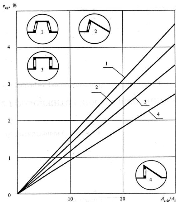
Рис. 28. График для определения среднего значения КЕО e_{cp} в общественных помещениях с фонарями. 1 – трапециевидный фонарь; 2 – шед, имеющий наклонное остекление; 3 – прямоугольный фонарь; 4 – шед, имеющий вертикальное остекление.
