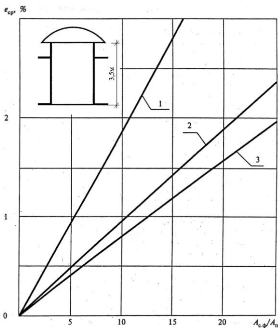
Рис. 27. График для определения среднего значения КЕО e_{cp} в общественных помещениях с шахтными фонарями диффузного света с глубиной светопроводной шахты 3,50м и размерами в плане, м: 1 - 2,9х5,9; 2 - 2,7х2,7; 2,9х2,9; 1,5х5,9; 3 - 1,5х1,7.
