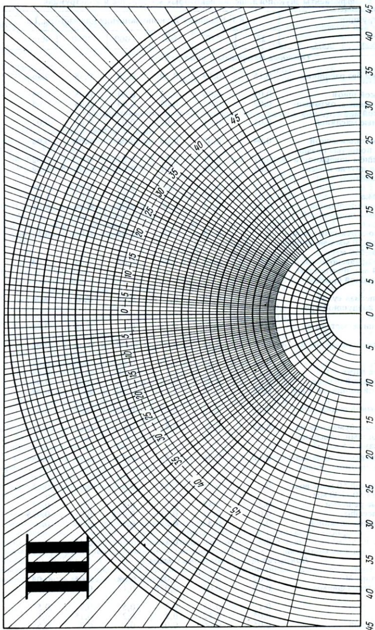
Рис. 38. График III А. М. Данилюка (НИИСФ) – с учетом q для систем верхнего света
