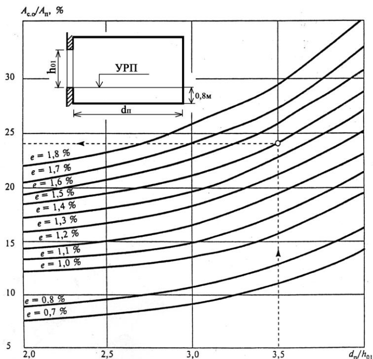
Рис. 24. График для определения относительной площади световых проемов A_{с.о}/A_n при боковом освещении школьных классов
