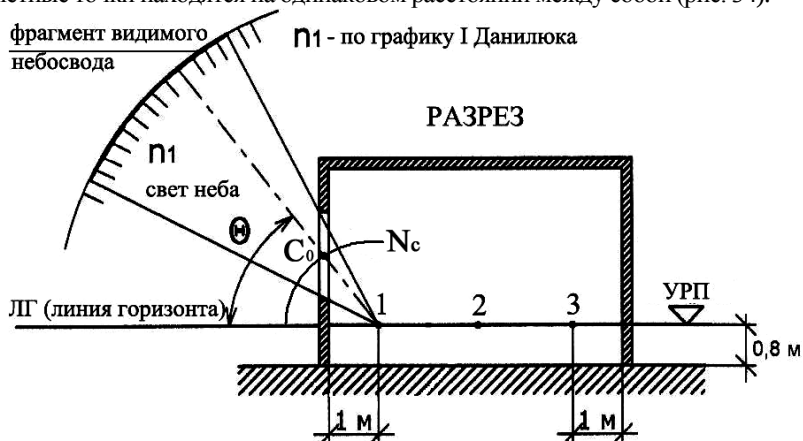
Рис. 34. Пример нахождения расчетных точек на УРП (или РП) величины n_1 , угла \theta и полуокружности N_c на графике I при открытом небосводе в плоскости характерного разреза помещения.
