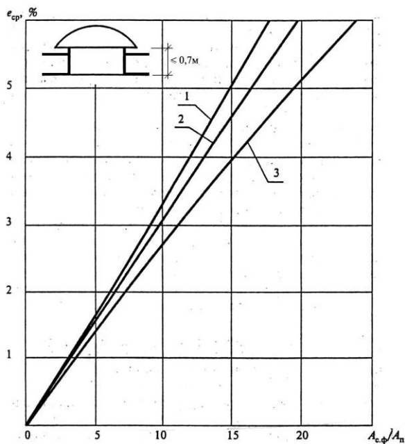
Рис. 25. График для определения среднего значения КЕО e_{cp} в помещениях с зенитными фонарями с глубиной проема до 0,7 м и размерами в плане, м: 1 - 2,9x5,9; 2 - 2,7x2,7; 2,9x2,9; 1,5x5,9; 3 - 1,5x1,7.
