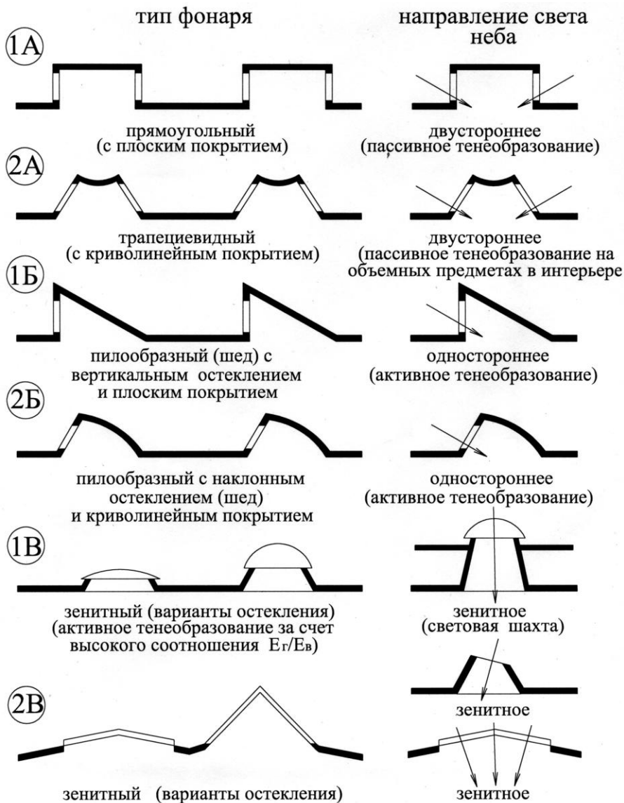
Рис.3. Классификация типов фонарей: А – П-образные, Б – пилообразные («шеды»), В – зенитные (точечные или линейные).
