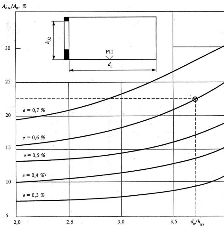
Рис. 22. График для определения относительной площади световых проемов A_{c.o.}/A_n при боковом освещении жилых помещений
