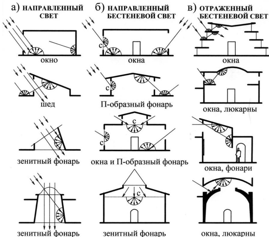
Рис.9. Классификация приемов естественного освещения по характеру светораспределения (с – светорассеивающее стекло).
