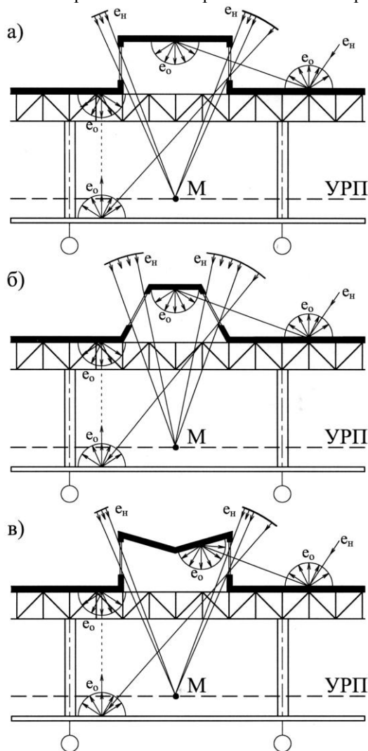
Рис. 5. Фонари-надстройки (однотипные П-образные): а – прямоугольные; б – трапециевидные; в - М-образные. Наклон стекол и форма покрытия фонаря могут варьироваться в зависимости от архитектурного решения.
