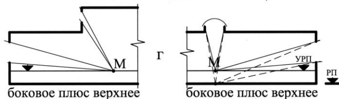
Рис.1. Схемы естественного освещения:
