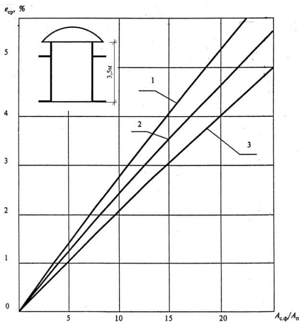
Рис. 26. График для определения среднего значения КЕО e_{cp} в общественных помещениях с шахтными фонарями с глубиной светопроводной шахты 3,50м и размерами в плане, м: 1 - 2,9x5,9; 2 - 2,7x2,7; 2,9x2,9; 1,5x5,9; 3 - 1,5x1,7.
