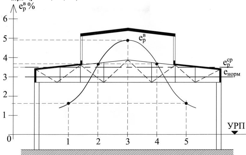
Рис. 44. Пример построения графика КЕО по результатам расчета верхнего естественного освещения (из табл. 16), если в тт. 1 и 5 e_p^B = 1,6\% , в тт. 2 и 4 e_p^B = 3,7\% , в т. 3 e_p^B = 4,9\% ; тогда e_{p\text{cp}} = (0,8 + 3,7 + 4,9 + 3,7 + 0,8) \approx 3,5\% .
