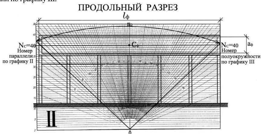
Рис. 43. Определение количества лучей n_2 , проходящих через световые проемы (фонари) на продольном разрезе помещения при верхнем освещении, по графику II.
