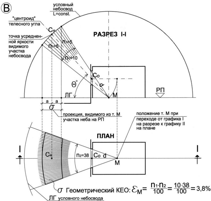
Рис. 32. Применение закона проекции вектора телесного угла в проверочных расчетах естественного освещения помещений на их ортогональных проекциях (разрез и план) с использованием графиков Данилюка.
