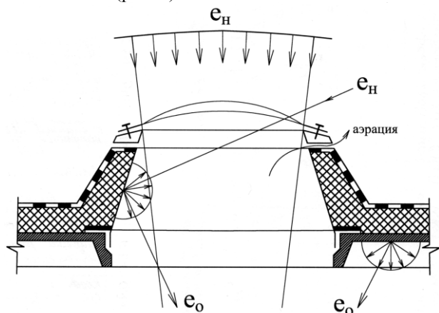
Рис. 7. Зенитные точечные фонари (купола с относительно глубокими шахтами-стаканами).
