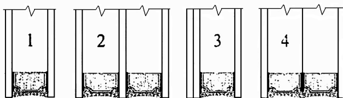
Рис. 13. Клееные стеклопакеты различной конструкции:
