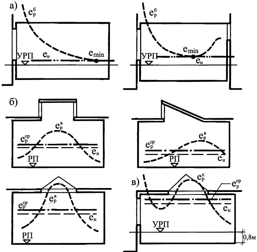
Рис. 20. Системы естественного освещения помещений и нормируемые значения КЕО (см. рис. 1).
