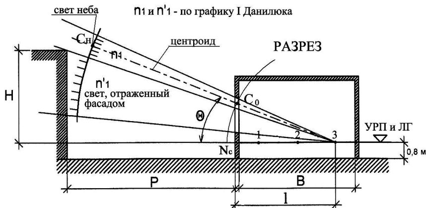
Рис. 35. Определение величины n_1 и n'_1 , а также угла \theta и полуокружности N_c при частично экранируемом небосводе*.
