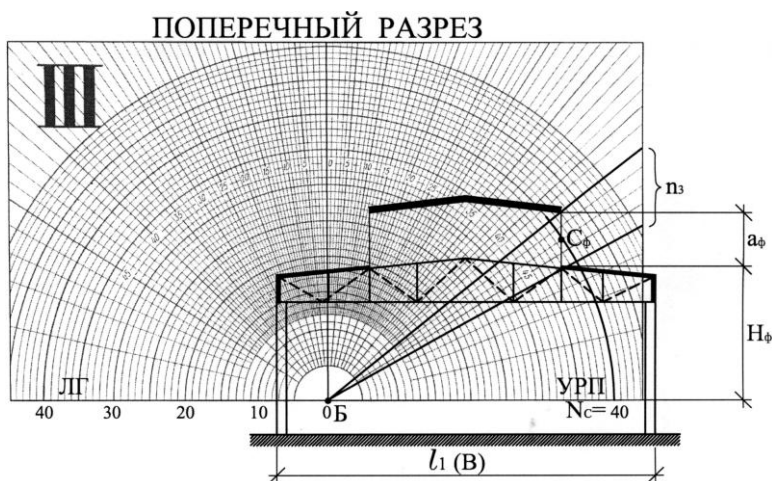
Рис. 42. Определение количества лучей n_3 , проходящих в расчетную точку Б через световые проемы (фонари) на поперечном разрезе помещения при верхнем освещении по графику III.
