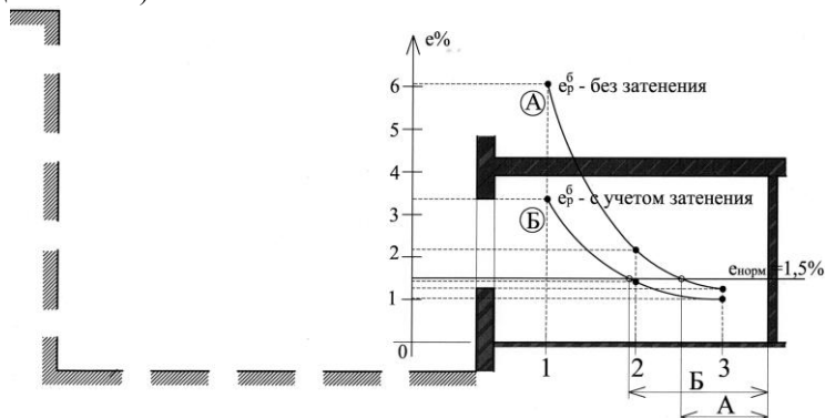
Рис. 41. Пример построения графиков КЕО при боковом свете по результатам расчета при отсутствии затенения (вариант А) и с учетом затенения (вариант Б) помещения противостоящим зданием:
