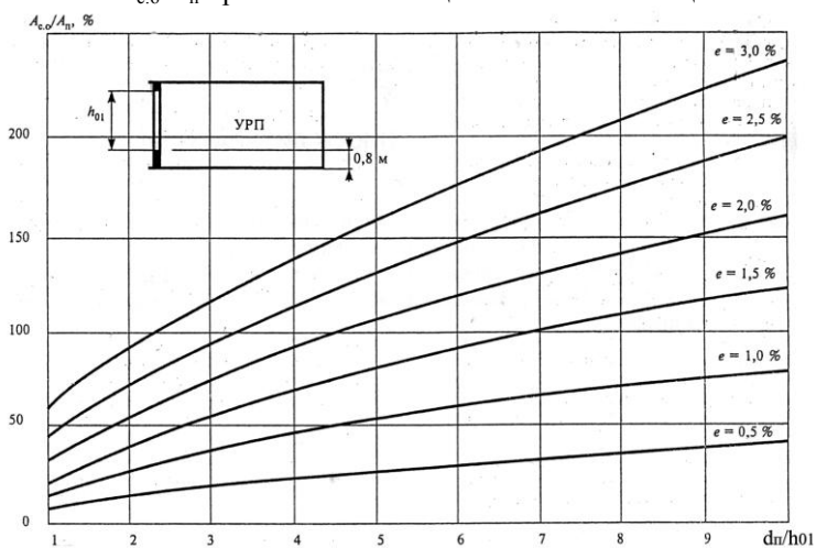
Рис. 23. График для определения относительной площади световых проемов A_{c.o.}/A_n при боковом освещении помещений общественных зданий
